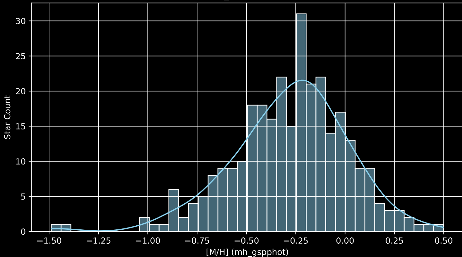
GALAH DR4 Field: [6963] [M/H] (mh_gspphot) (n= 299)
