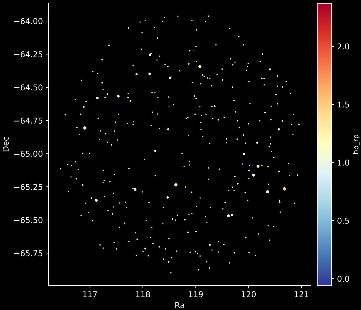
GALAH DR4 Field: [6963] Stars: 300
