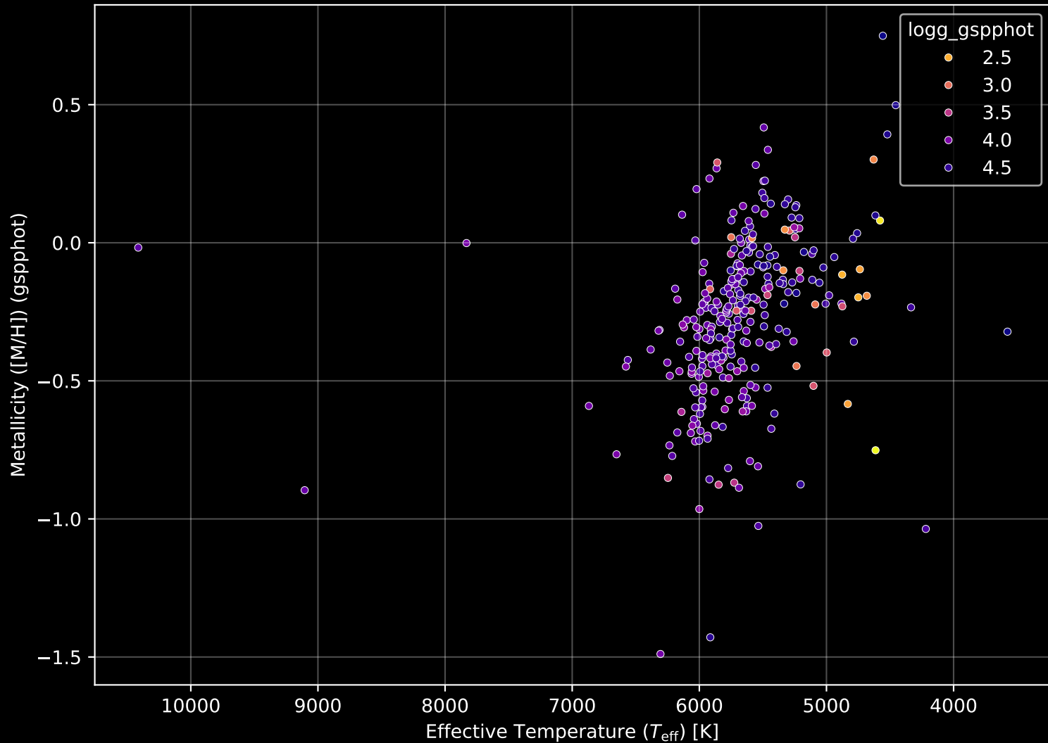
GALAH DR4 Field: [6963] Stellar Population Parameters (n= 300)
