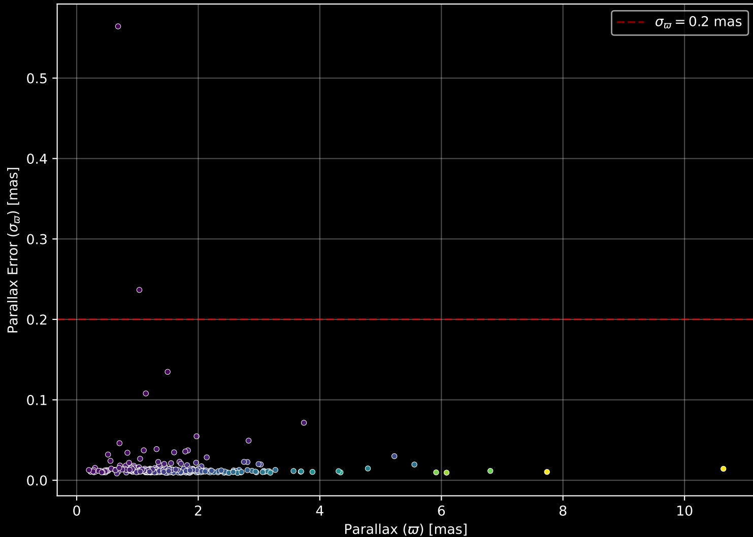
GALAH DR4 Field: [6963] Parallax Quality (n= 300)
